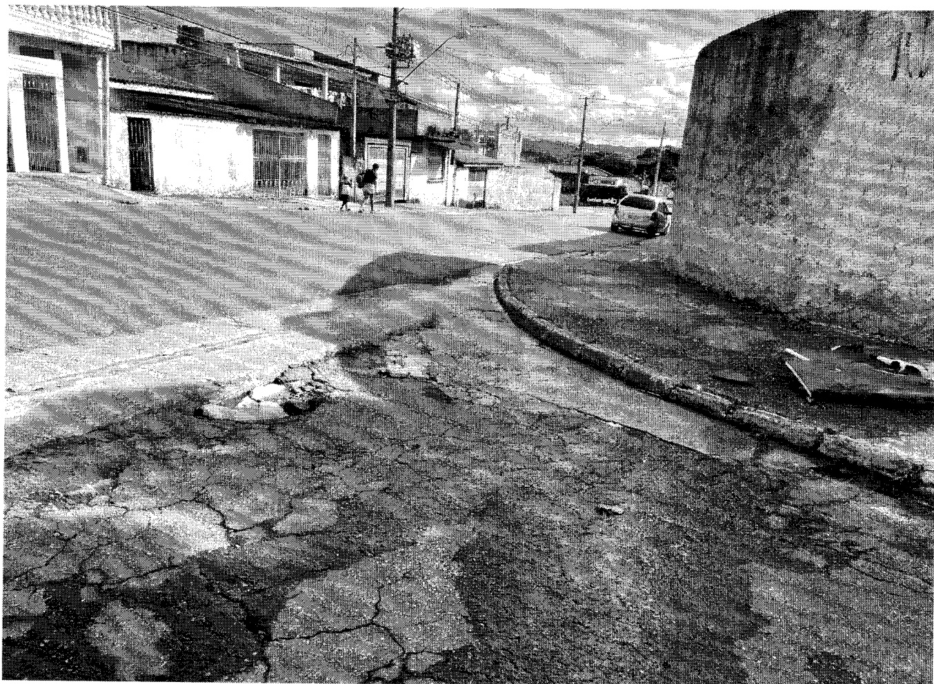
Manutenção Asfáltica em toda extensão asfáltica na Rua Embiruçu. Jd. Planalto - Mogi das Cruzes
